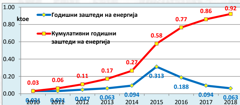
График 6.2.2.1: Енергетски заштеди што ги произведува проектот за јавно осветлување 7
