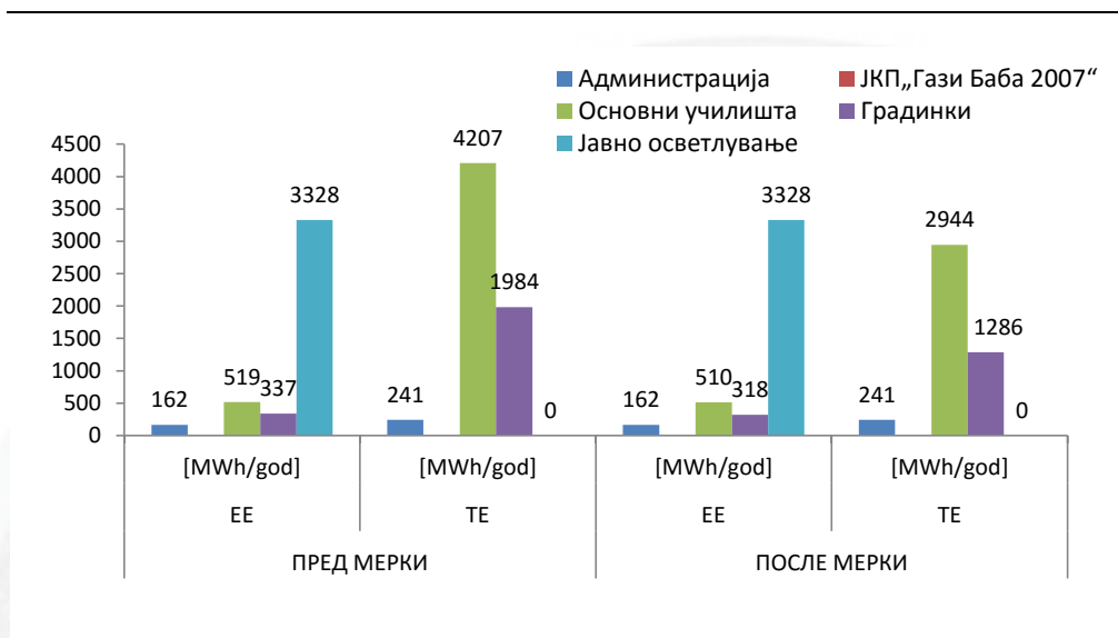
График 6.2.6.2: Потенцијал за енергетска ефикасност за топлинска и електрична енергија во општинските објекти и јавното осветление
