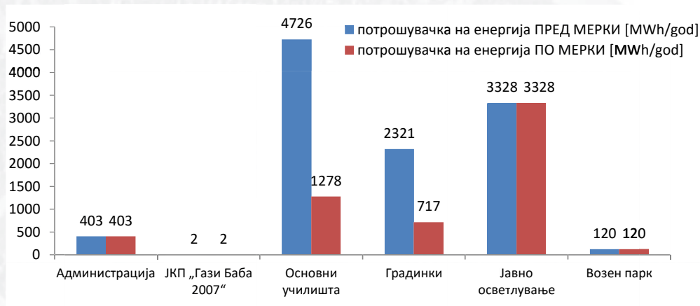
График 6.1.2: Потенцијал за енергетска ефикасност во општинските објекти и јавното осветление
