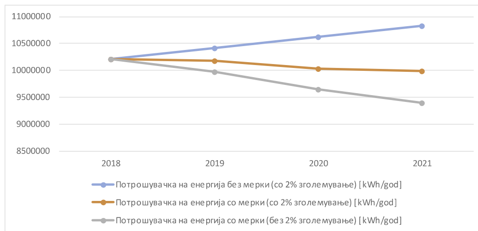
Слика Проценет развој на потрошувачката на енергија во период од 201 до 202 година
