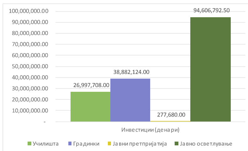
Слика Инвестиции согласно вкупниот потенцијал за енергетска ефикасност во Општина Гази Баба
