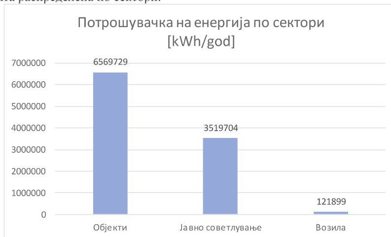
Слика Просечна потрошувачка на енергија во Општина Гази Баба
