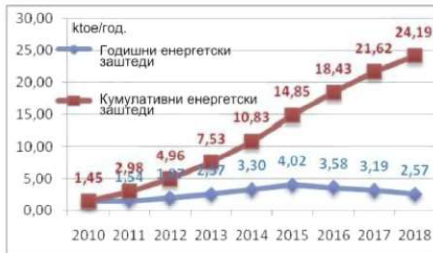
Слика Енергетски заштеди што ги произведува комерцијалниот и услужниот сектор според Националниот акциски план за енергетска ефикасност на Македонија
