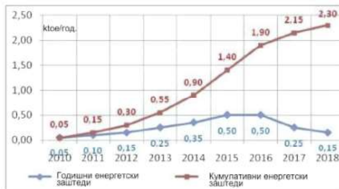
Слика Енергетски заштеди што ги произведува подобреното енергетско управување во општините
